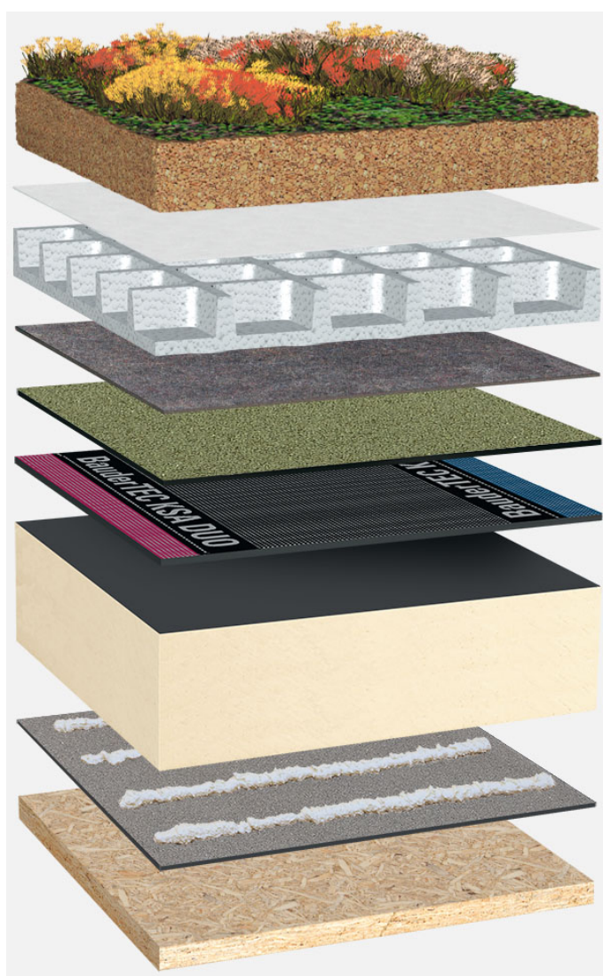
Systemowy układ warstw: HG_PIR-FA_P_01_G75
