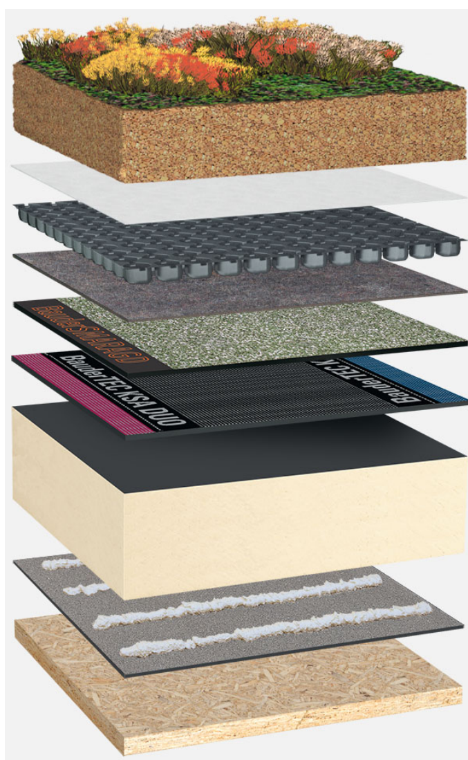
Systemowy układ warstw: HG_PIR-FA_S_01_G125
