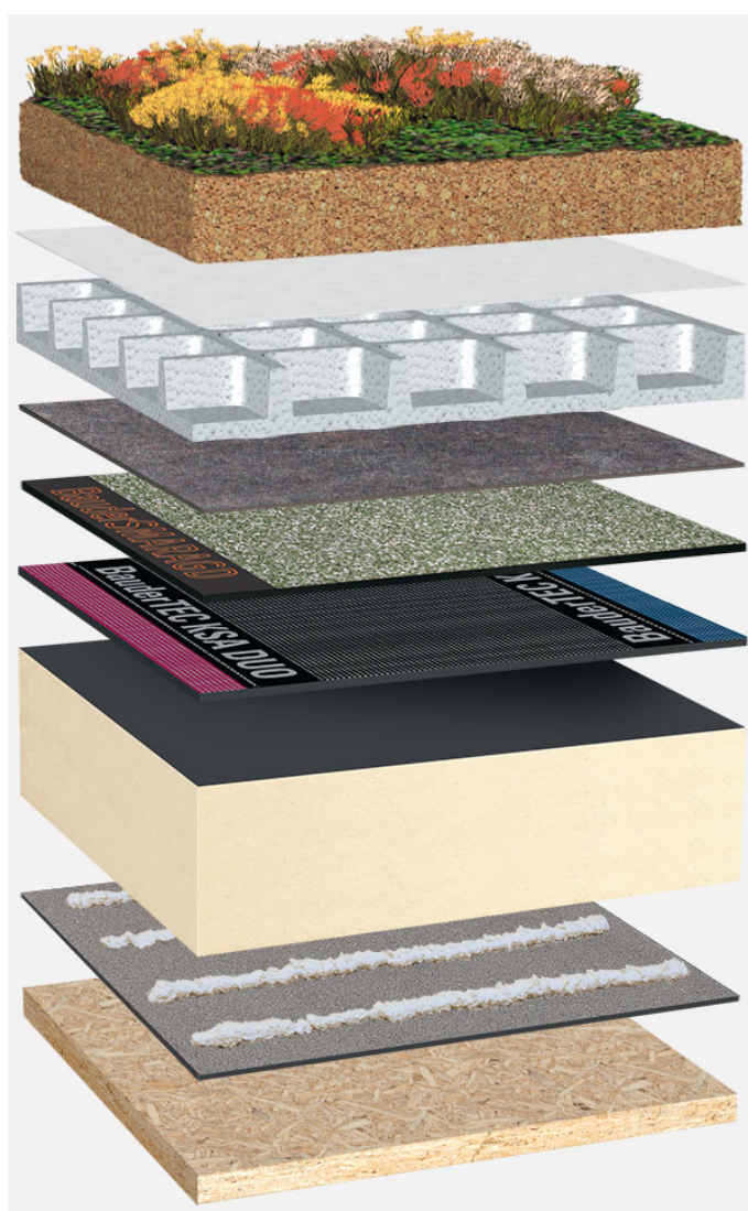
Systemowy układ warstw: HG_PIR-FA_S_01_G75
