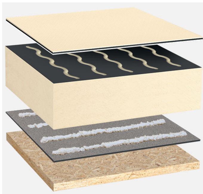
Systemowy układ warstw: HG_PIR-FA_TV_01
