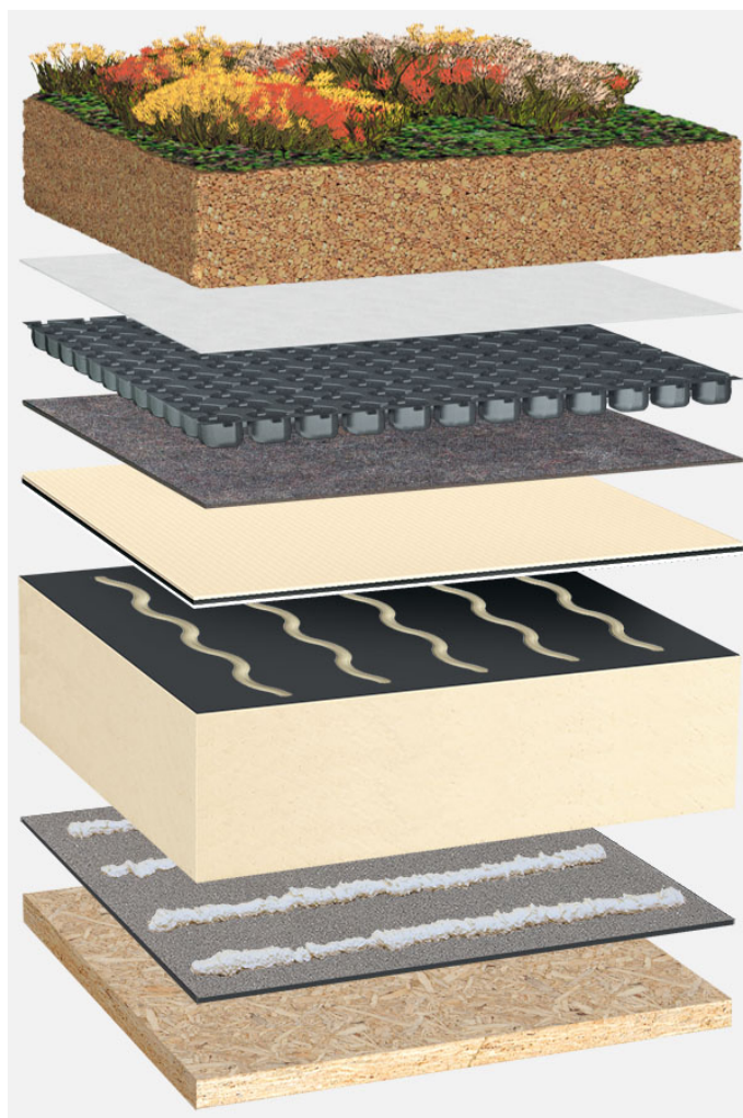
Systemowy układ warstw: HG_PIR-FA_TV_01_G125
