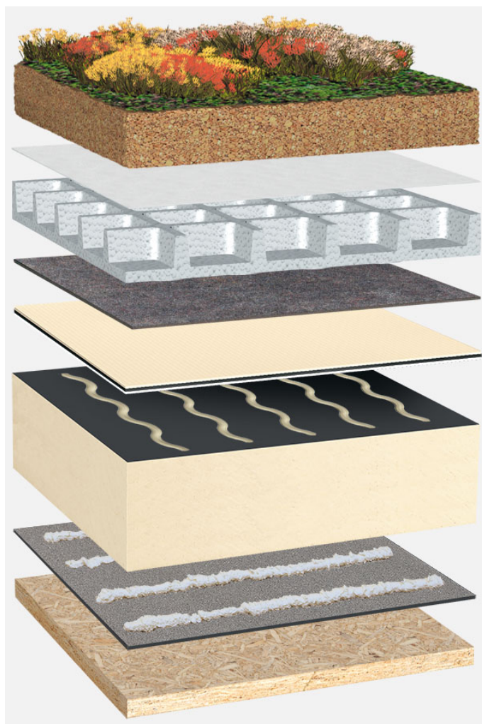
Systemowy układ warstw: HG_PIR-FA_TV_01_G75
