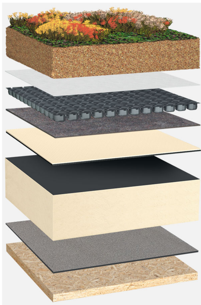
Systemowy układ warstw: HG_PIR-FA_T_01_G125
