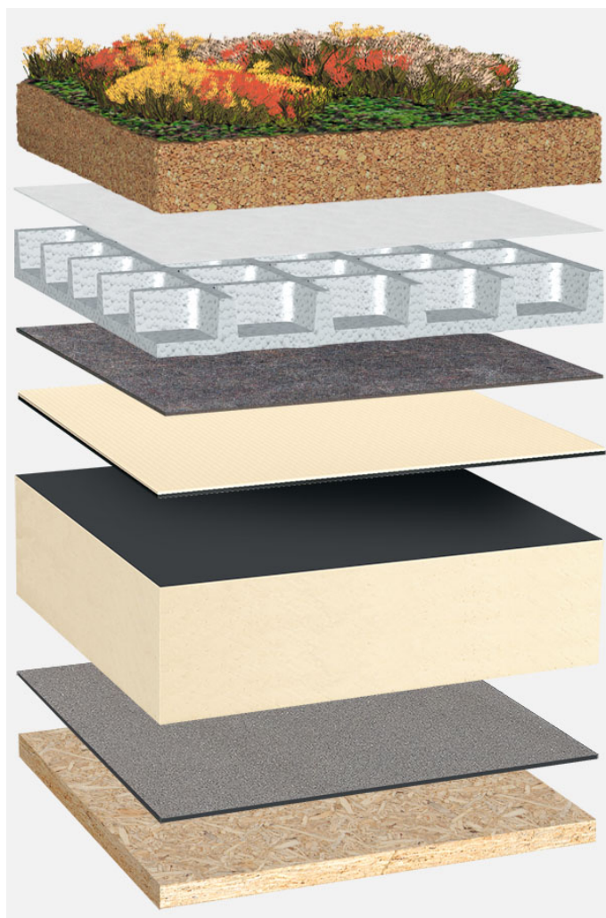
Systemowy układ warstw: HG_PIR-FA_T_01_G75
