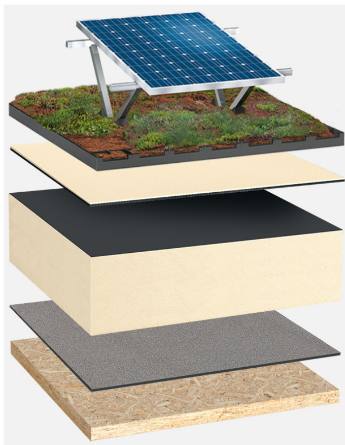
Systemowy układ warstw: HG_PIR-FA_T_01_PVGD
