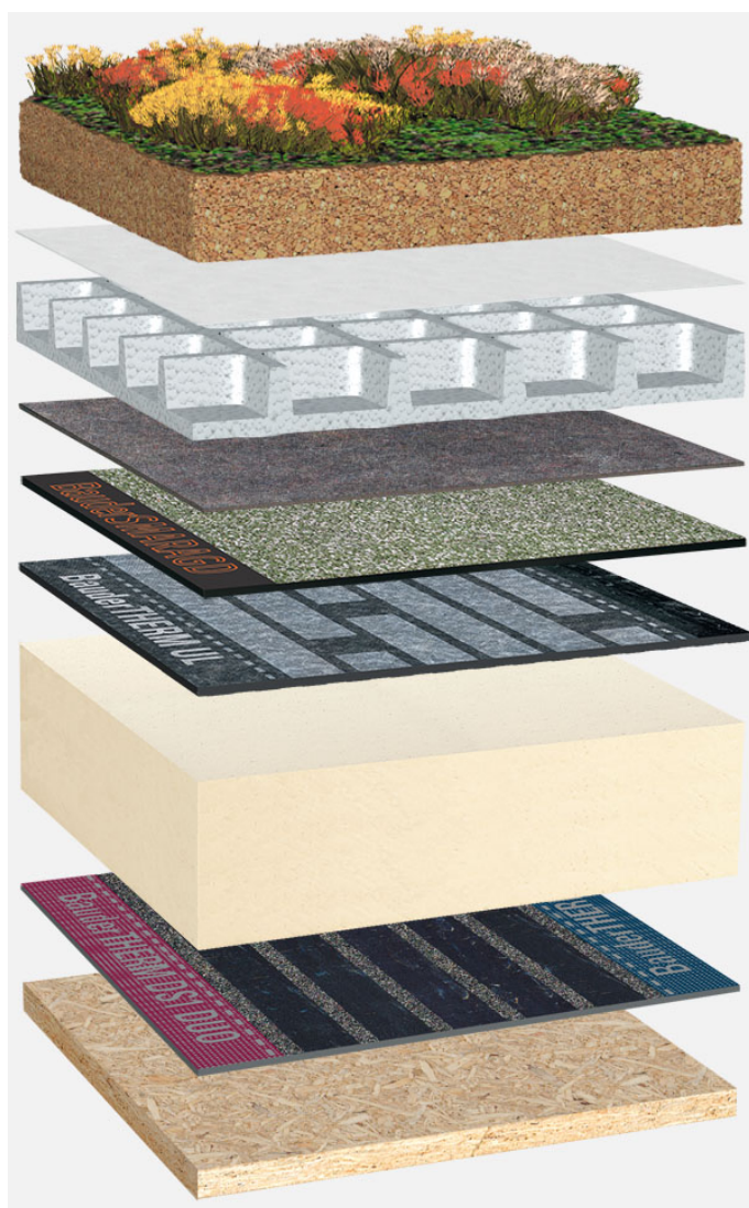
Systemowy układ warstw: HG_PIR-MF_S_01_G75
