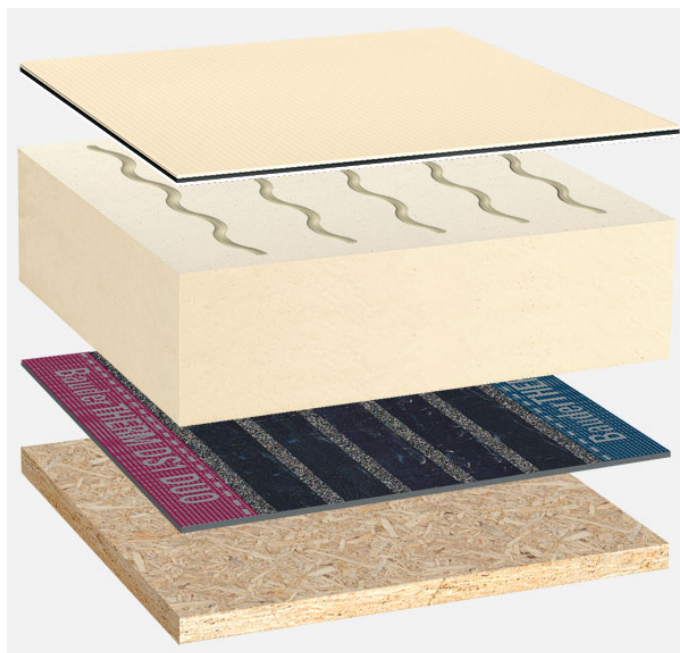
Systemowy układ warstw: HG_PIR-MF_TV_01
