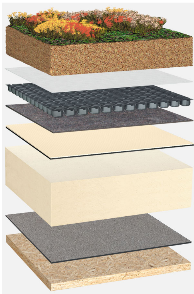
Systemowy układ warstw: HG_PIR-MF_T_01_G125
