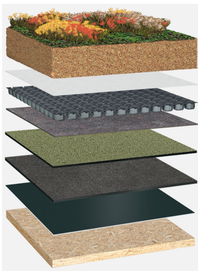
Systemowy układ warstw: HG_P_01_G125
