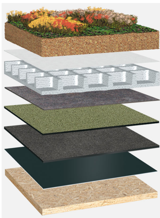
Systemowy układ warstw: HG_P_01_G75
