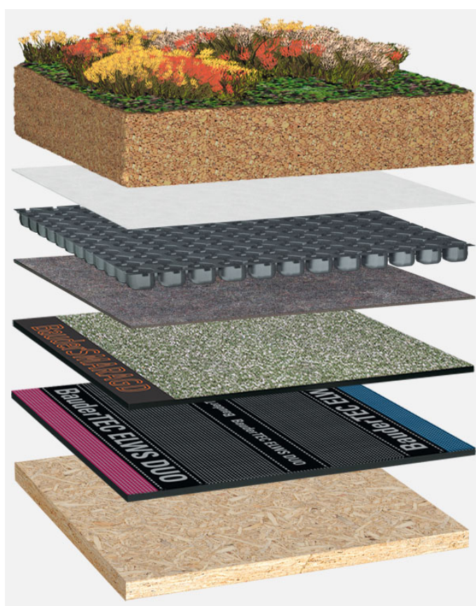
Systemowy układ warstw: HG_S_01_G125
