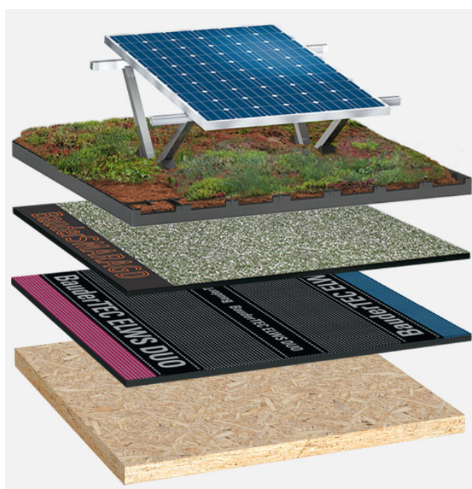
Systemowy układ warstw: HG_S_01_PVGD
