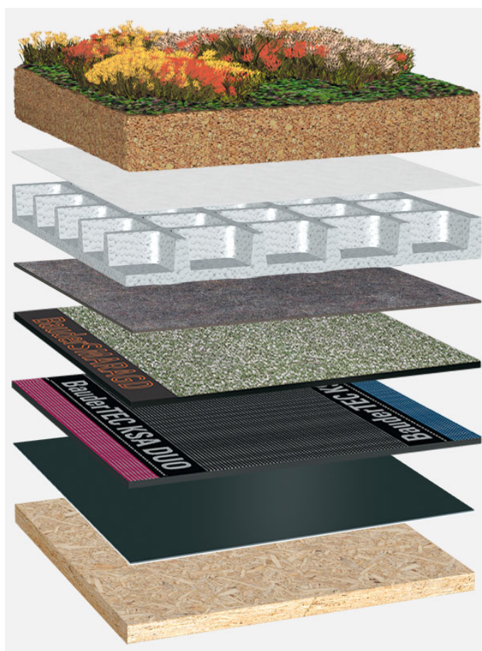
Systemowy układ warstw: HG_S_02_G75
