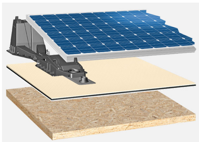
Systemowy układ warstw: HG_TV_01_PVFD
