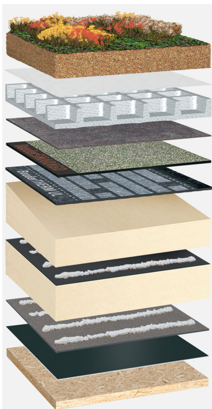
Systemowy układ warstw: HP_PIR-FA_PIR-TG_S_01_G75
