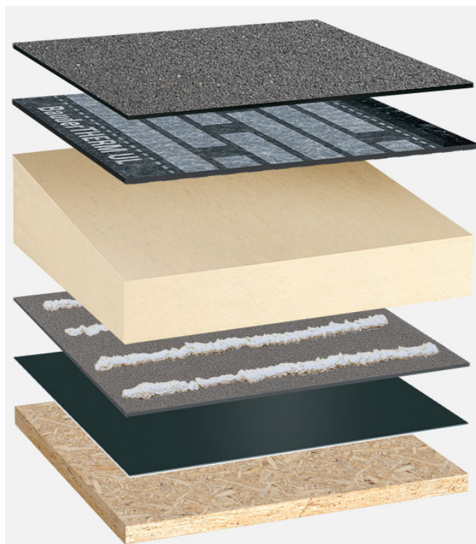
Systemowy układ warstw: HP_PIR-TG_B_01
