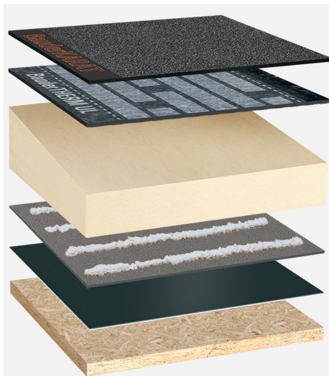
Systemowy układ warstw: HP_PIR-TG_K_01
