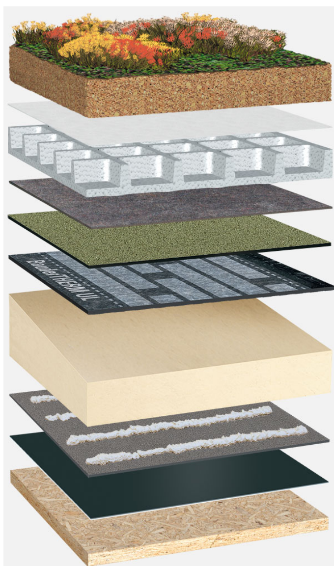
Systemowy układ warstw: HP_PIR-TG_P_01_G125
