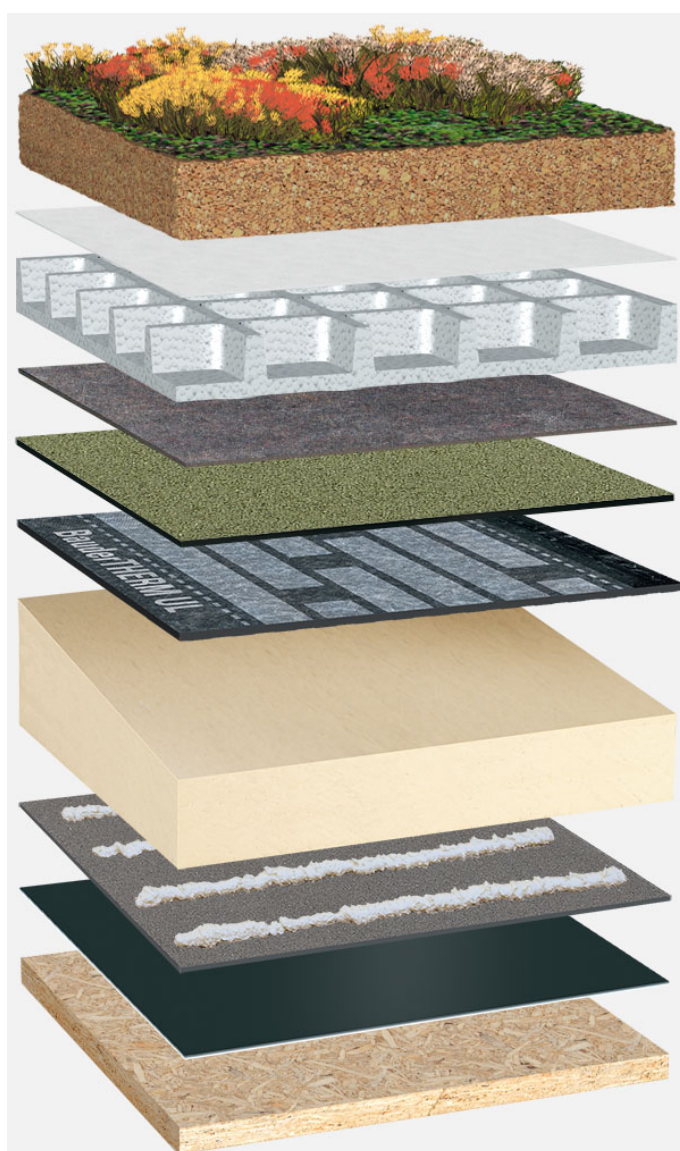
Systemowy układ warstw: HP_PIR-TG_P_01_G75
