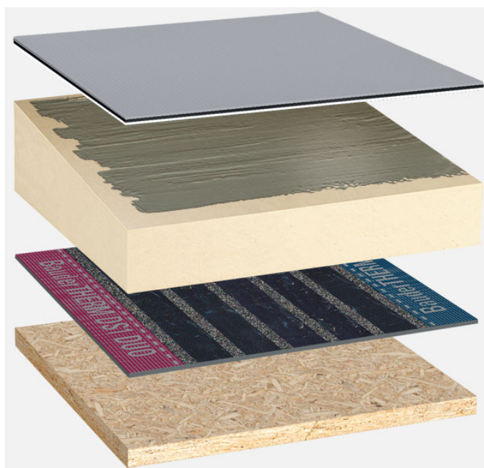
Systemowy układ warstw: HP_PIR-TG_SK_01
