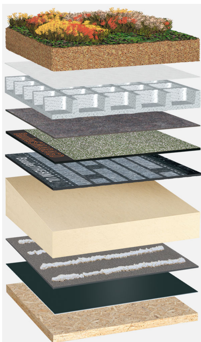
Systemowy układ warstw: HP_PIR-TG_S_01_G75
