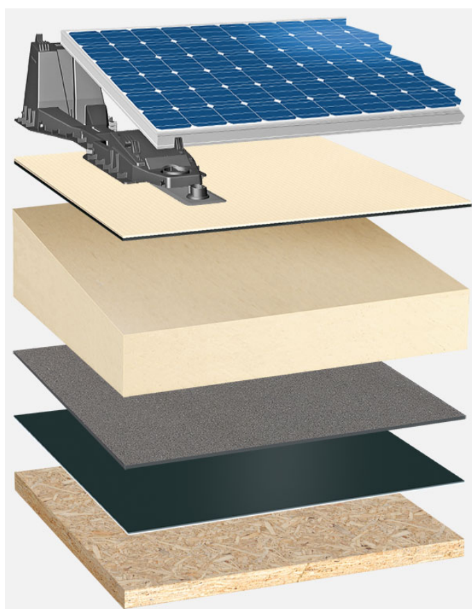
Systemowy układ warstw: HP_PIR-TG_T_01_PVFD
