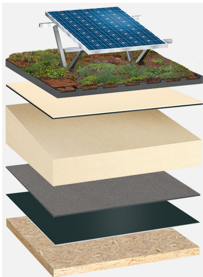
Systemowy układ warstw: HP_PIR-TG_T_01_PVGD
