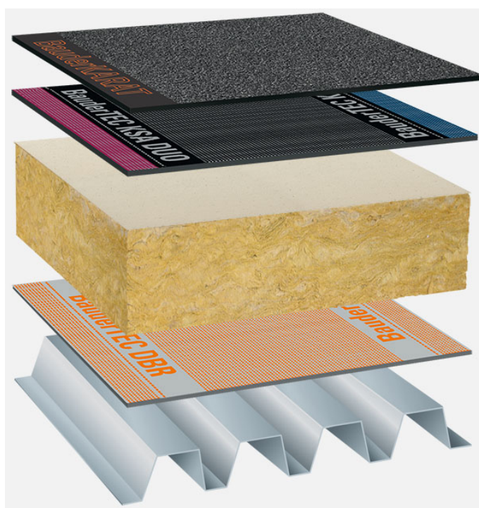
Systemowy układ warstw: IG_MIFA-P_K_01
