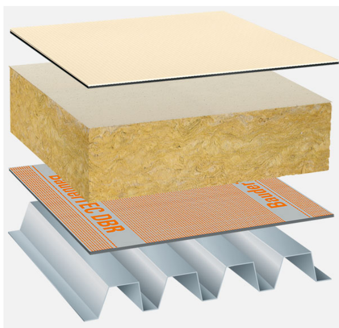
Systemowy układ warstw: IG_MIFA-P_T_01
