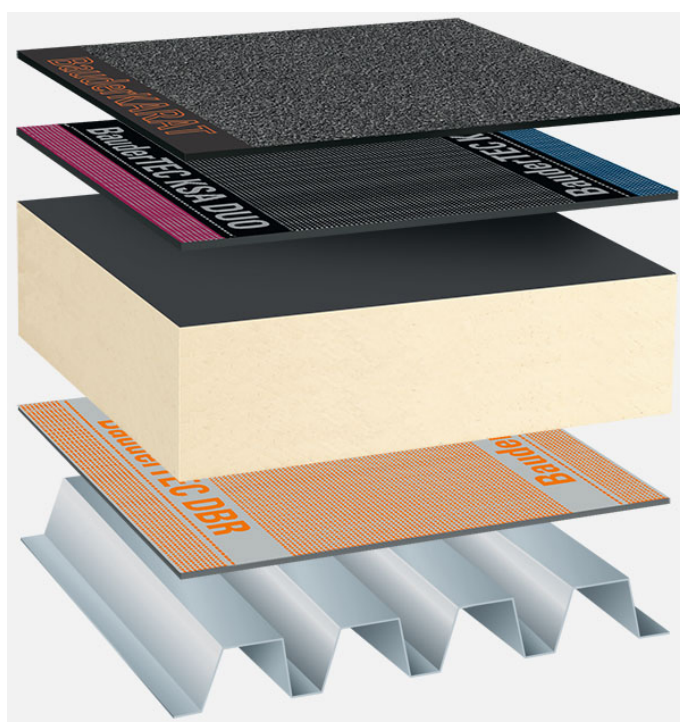
Systemowy układ warstw: IG_PIR-FA_K_01
