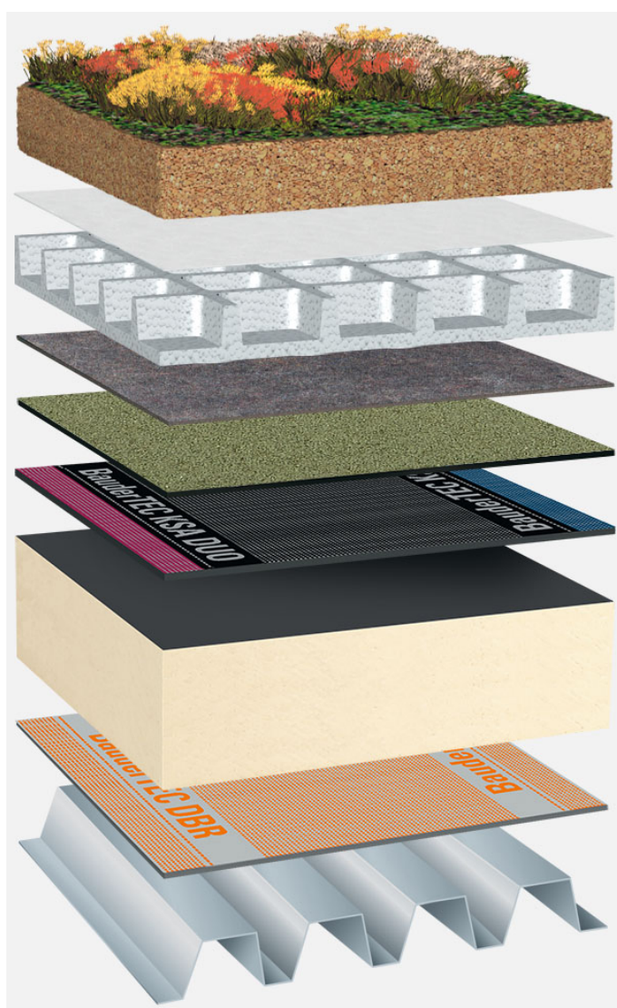
Systemowy układ warstw: IG_PIR-FA_P_01_G75
