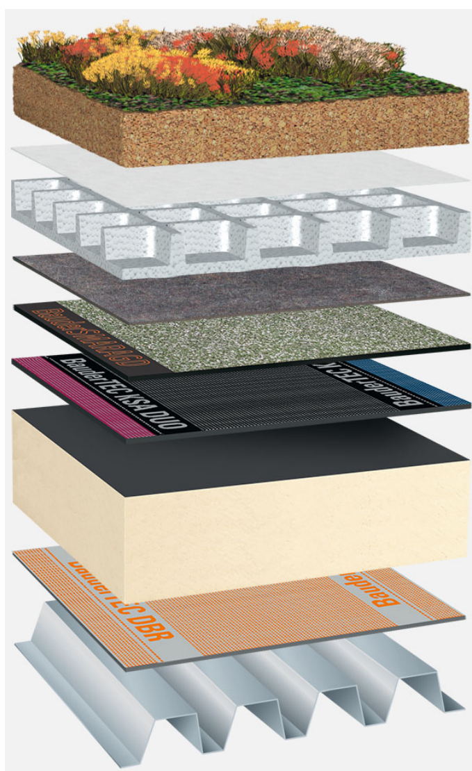
Systemowy układ warstw: IG_PIR-FA_S_01_G75
