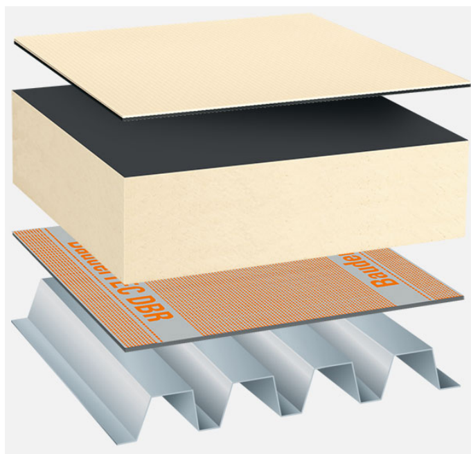
Systemowy układ warstw: IG_PIR-FA_T_01
