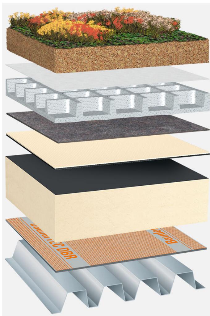
Systemowy układ warstw: IG_PIR-FA_T_01_G75
