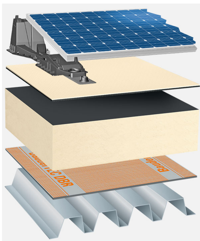
Systemowy układ warstw: IG_PIR-FA_T_01_PVFD
