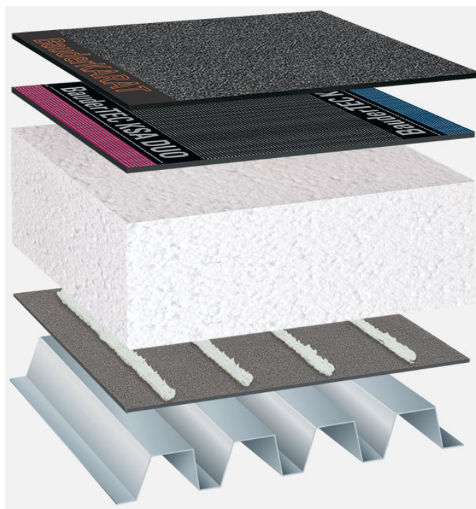
Systemowy układ warstw: TG_EPS-P_K_01
