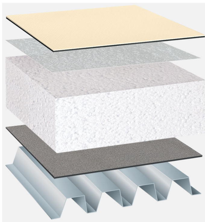
Systemowy układ warstw: TG_EPS-P_T_01
