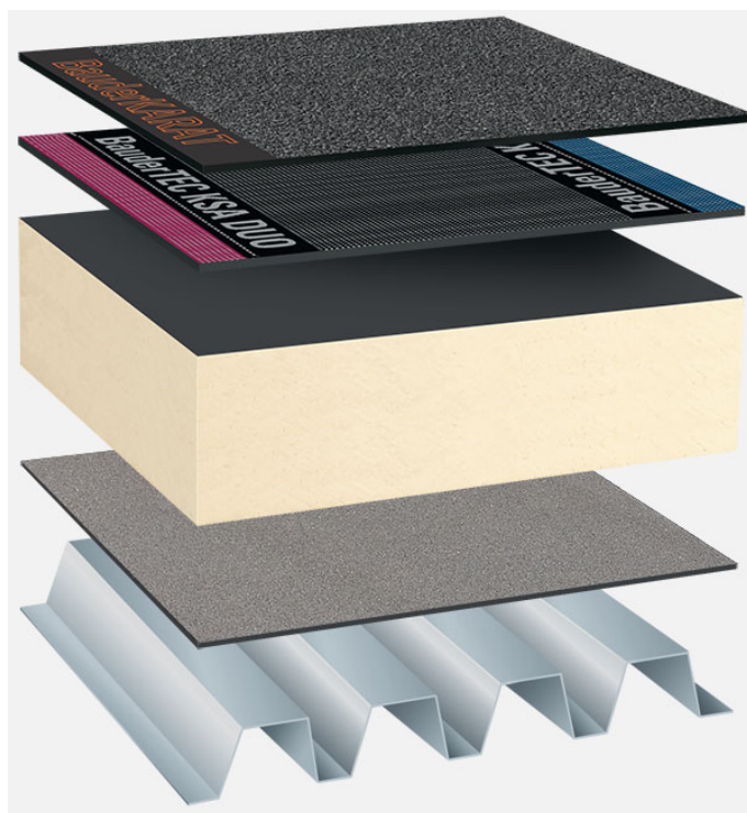
Systemowy układ warstw: TG_PIR-FA_K_01
