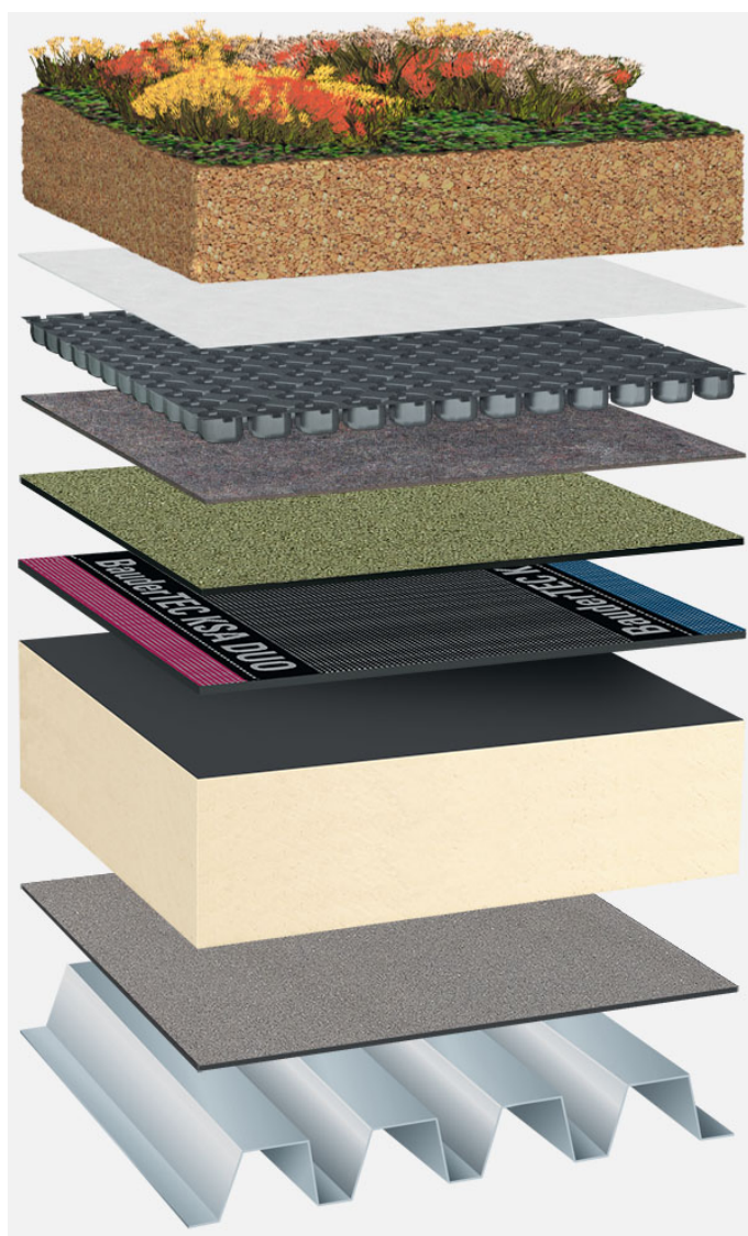
Systemowy układ warstw: TG_PIR-FA_P_01_G125
