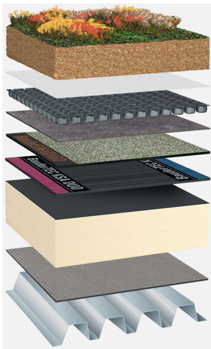
Systemowy układ warstw: TG_PIR-FA_S_01_G125
