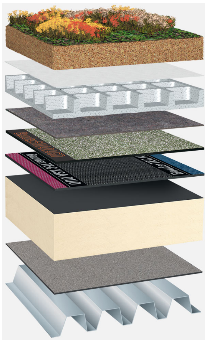
Systemowy układ warstw: TG_PIR-FA_S_01_G75
