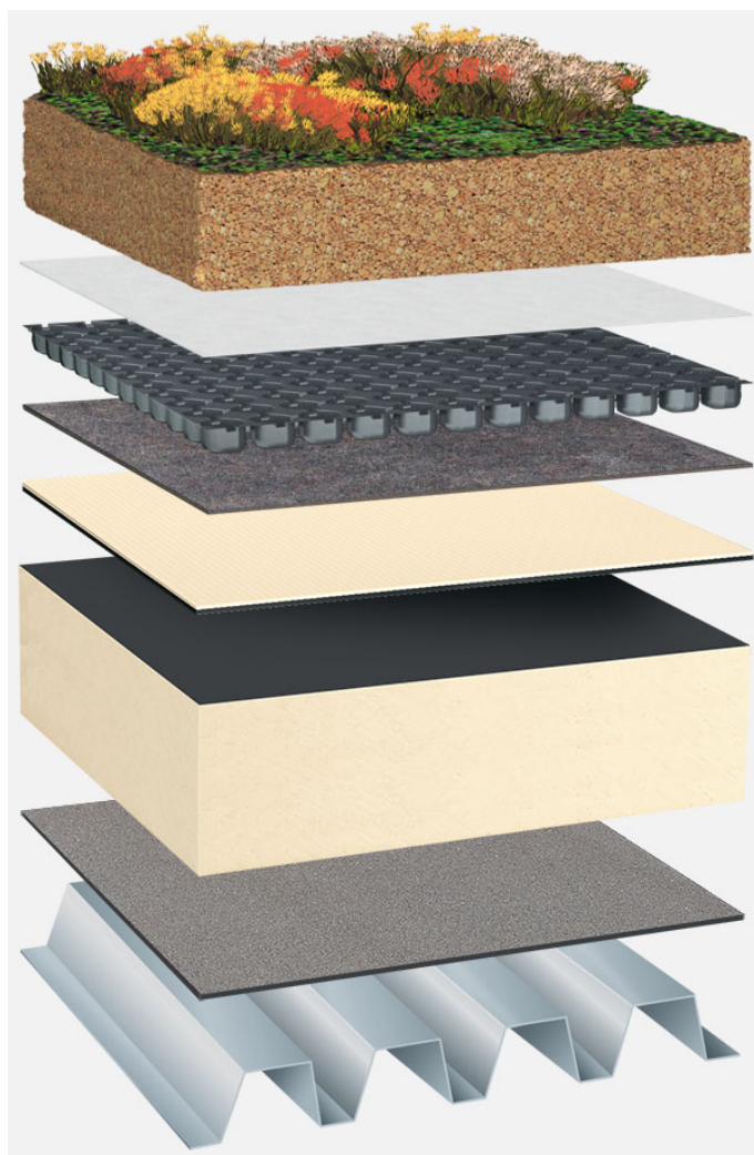
Systemowy układ warstw: TG_PIR-FA_T_01_G125
