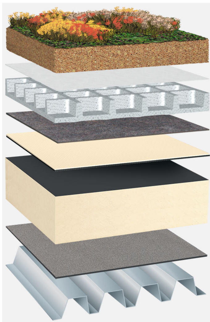
Systemowy układ warstw: TG_PIR-FA_T_01_G75
