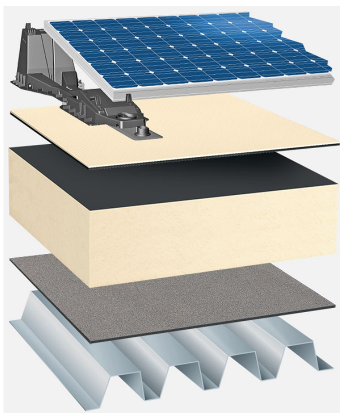
Systemowy układ warstw: TG_PIR-FA_T_01_PVFD
