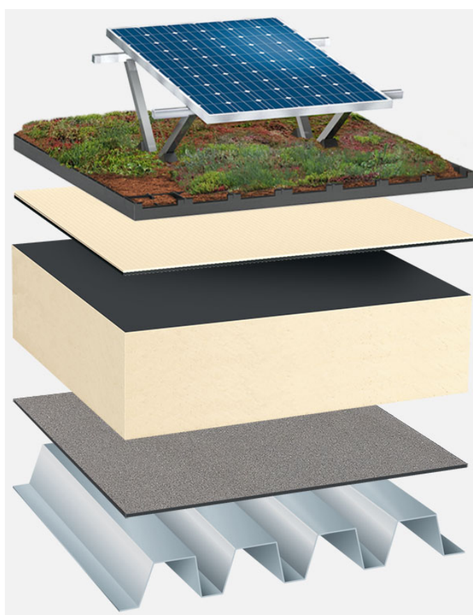
Systemowy układ warstw: TG_PIR-FA_T_01_PVGD
