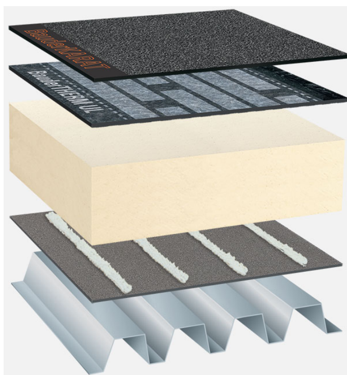
Systemowy układ warstw: TG_PIR-MF_K_01
