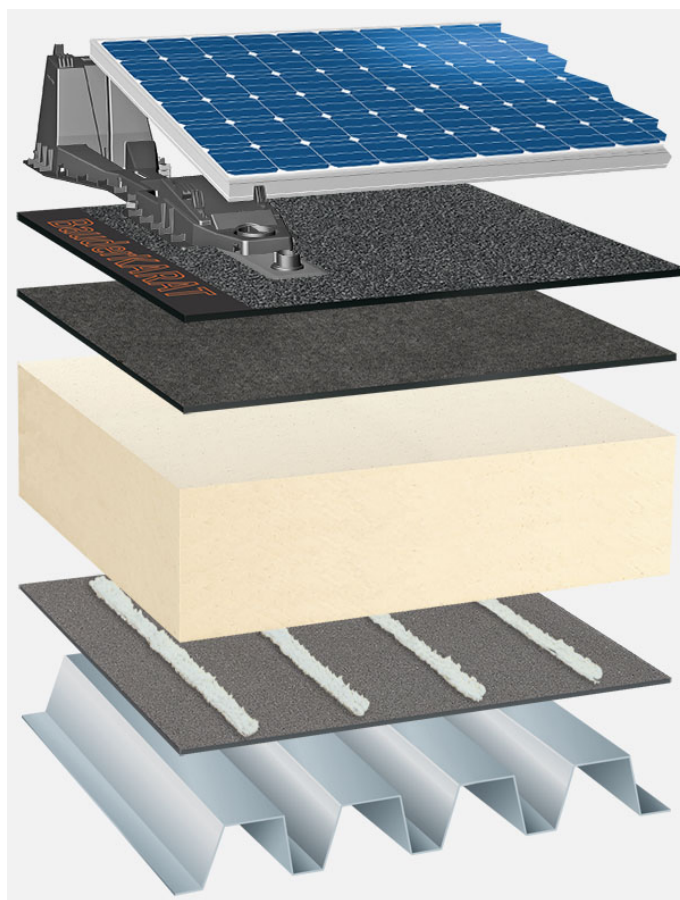
Systemowy układ warstw: TG_PIR-MF_K_01_PVFD
