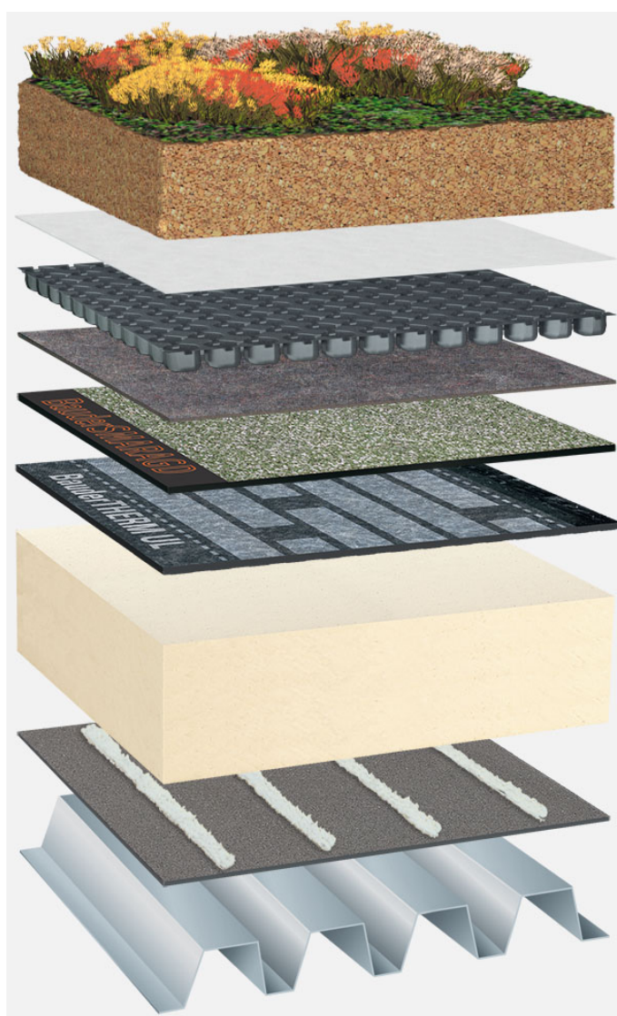
Systemowy układ warstw: TG_PIR-MF_S_01_G125
