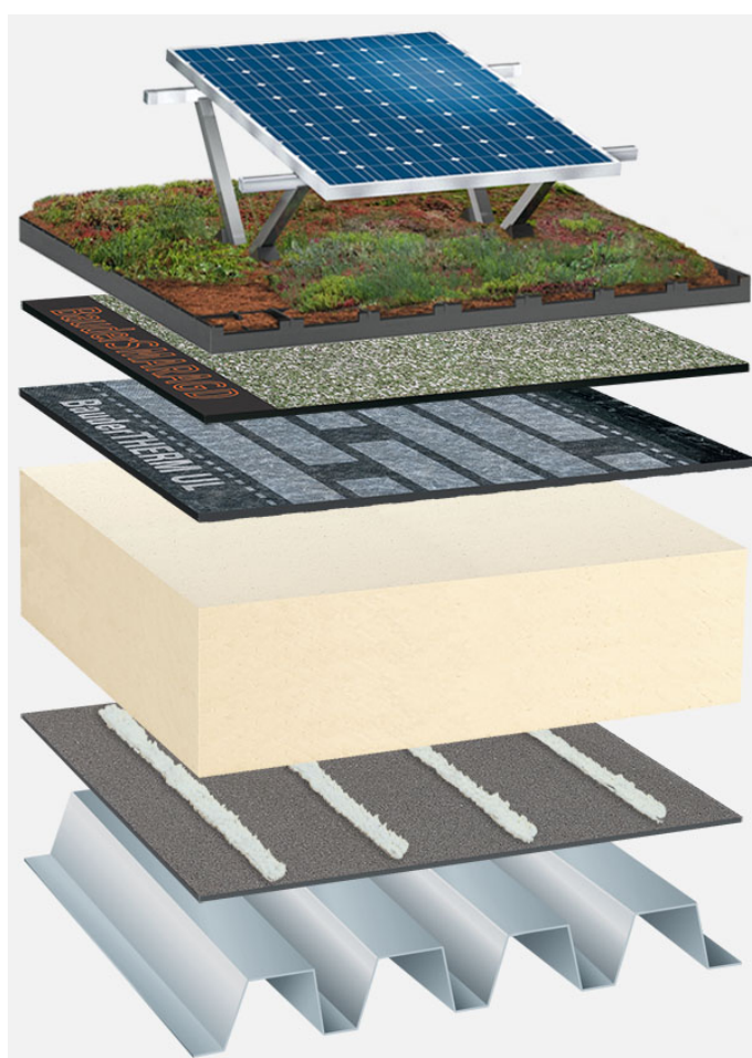
Systemowy układ warstw: TG_PIR-MF_S_01_PVGD
