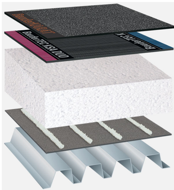
Systemowy układ warstw: TP_EPS-G_K_01
